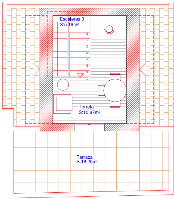
Planta Torre
