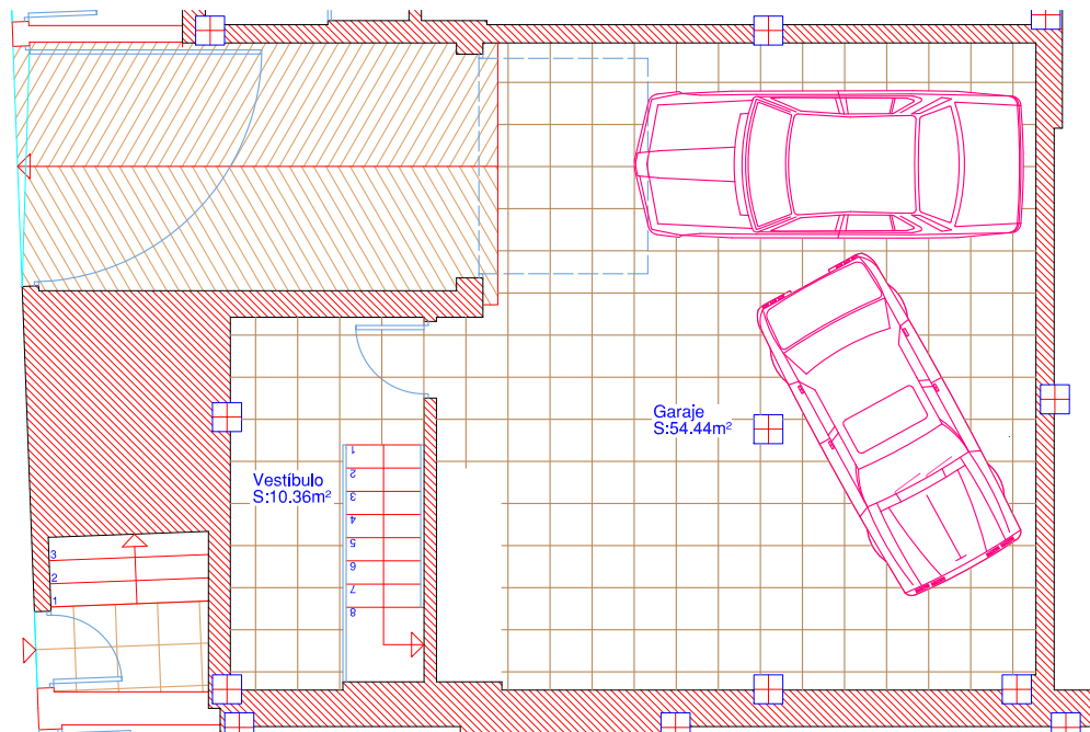
Planta Semisótano
