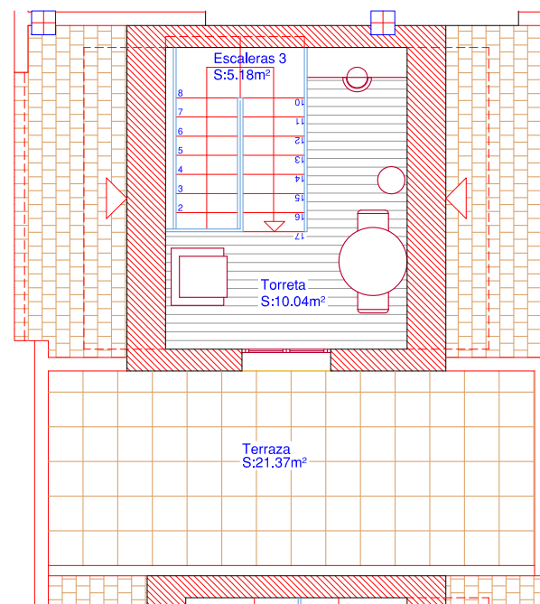
Planta Torreta
