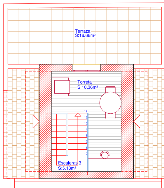
Planta Torreta
