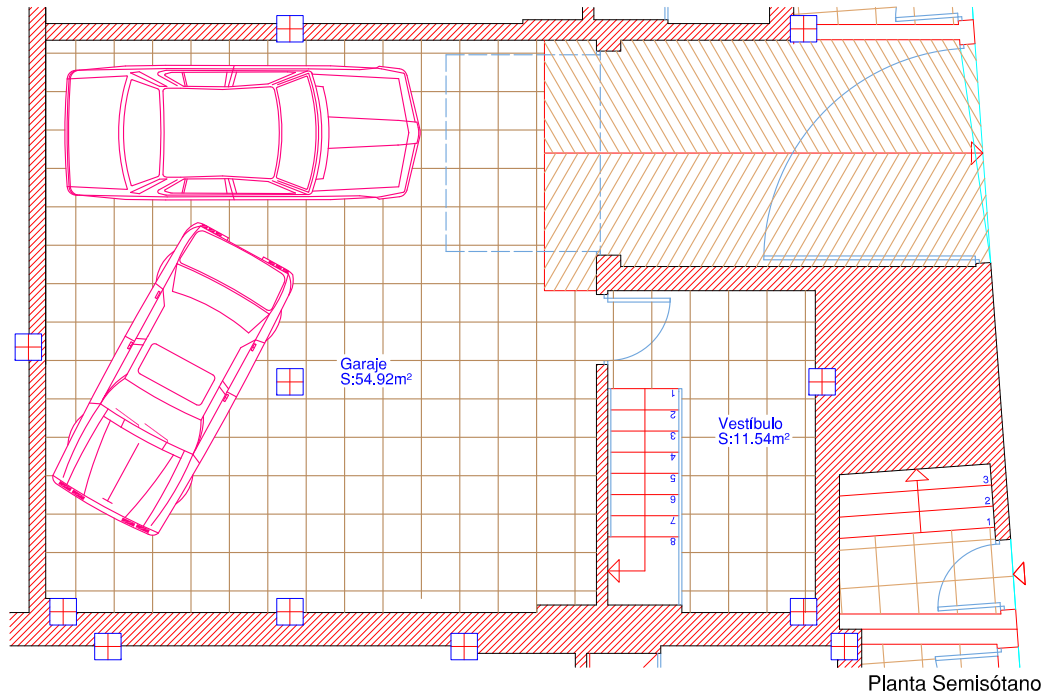
Planta Semisótano
