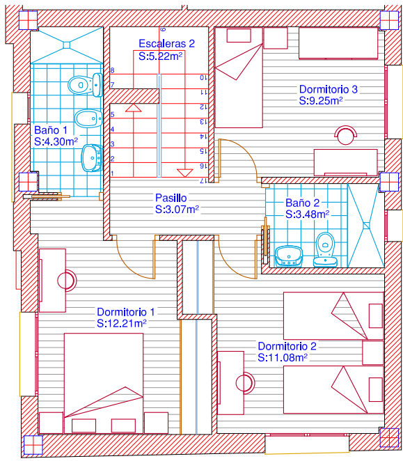
Planta Primera
