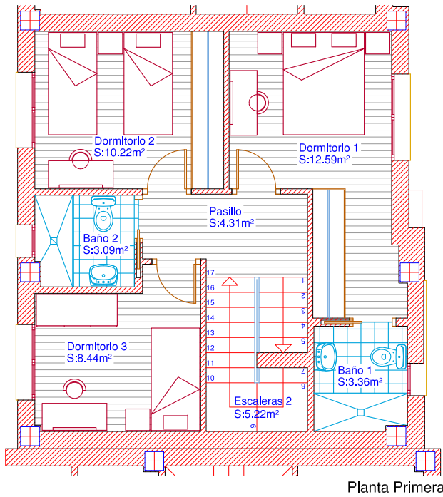
Planta Primera
