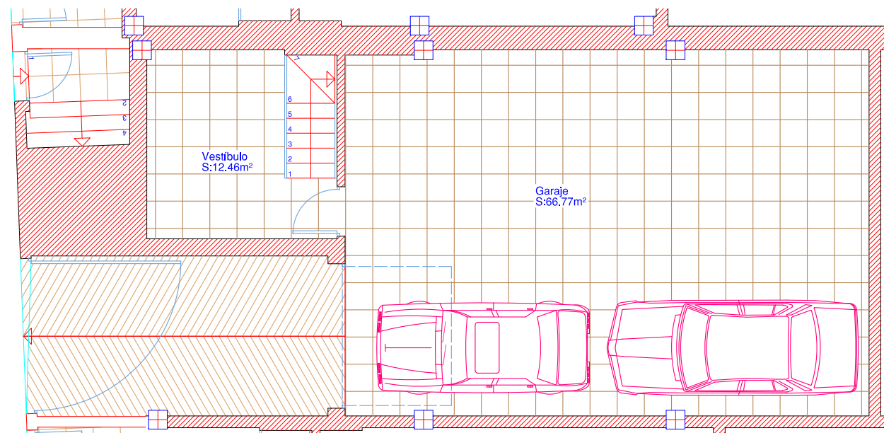
Planta Semisótano
