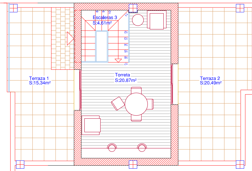
Planta Torreta
