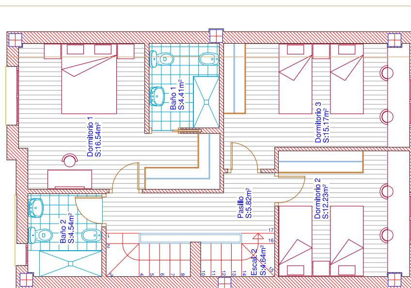
Planta Primera
