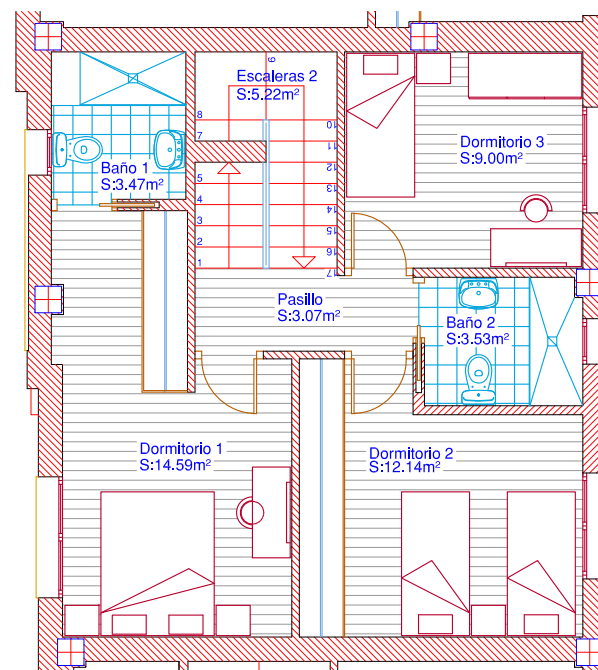
Planta Primera
