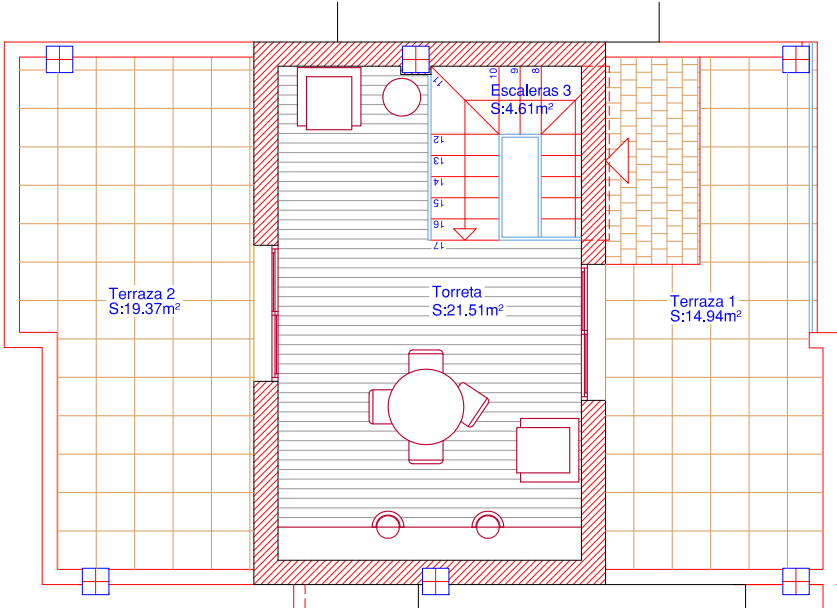
Planta Torreta
