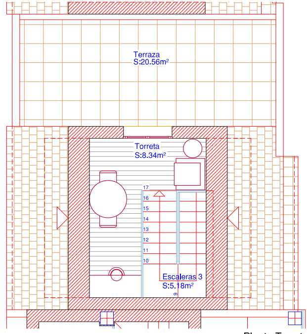
Planta Torreta
