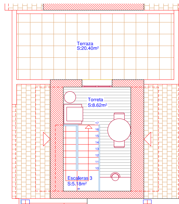
Planta Torre
