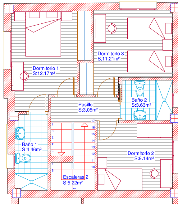
Planta Primera
