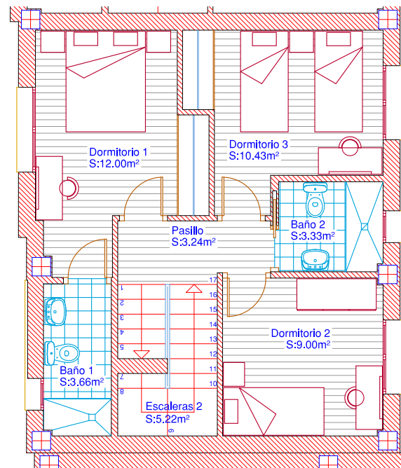
Planta Primera
