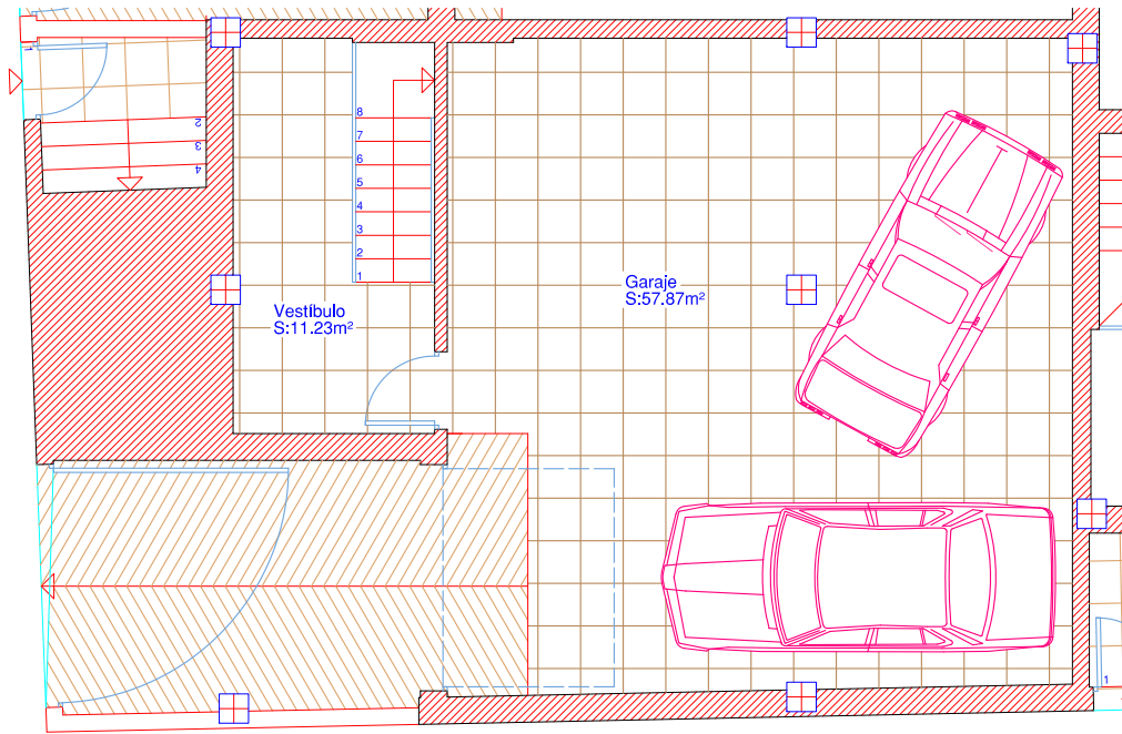
Planta Semisótano
