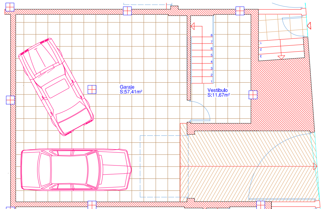
Planta Semisótano
