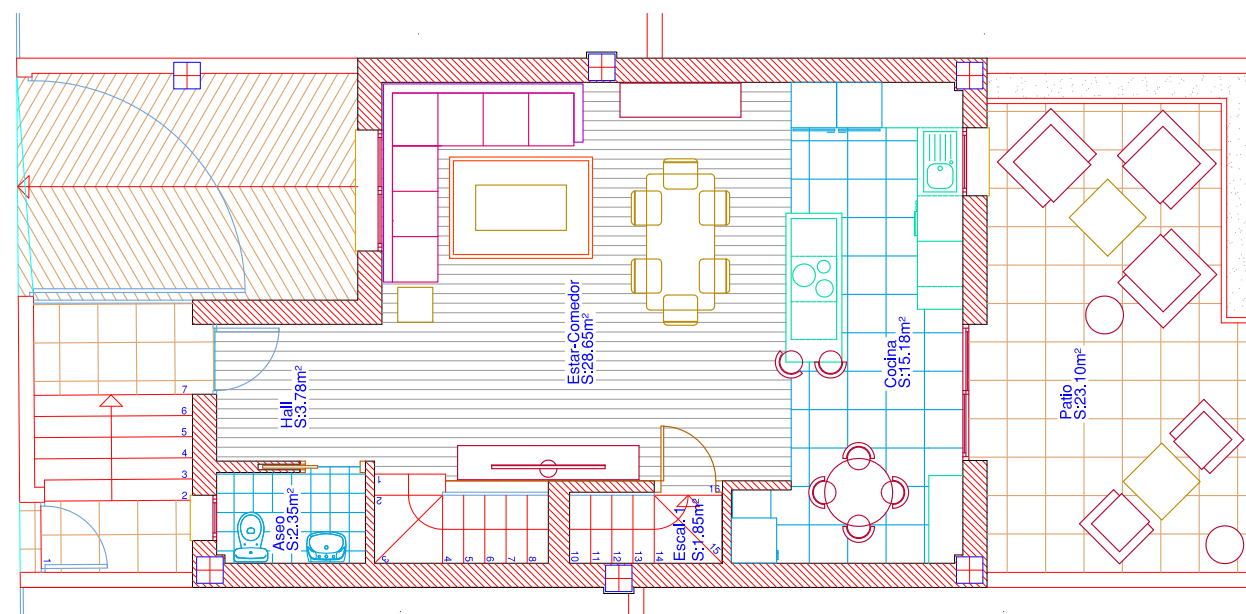
Planta Baja
