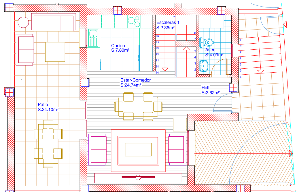
Planta Baja
