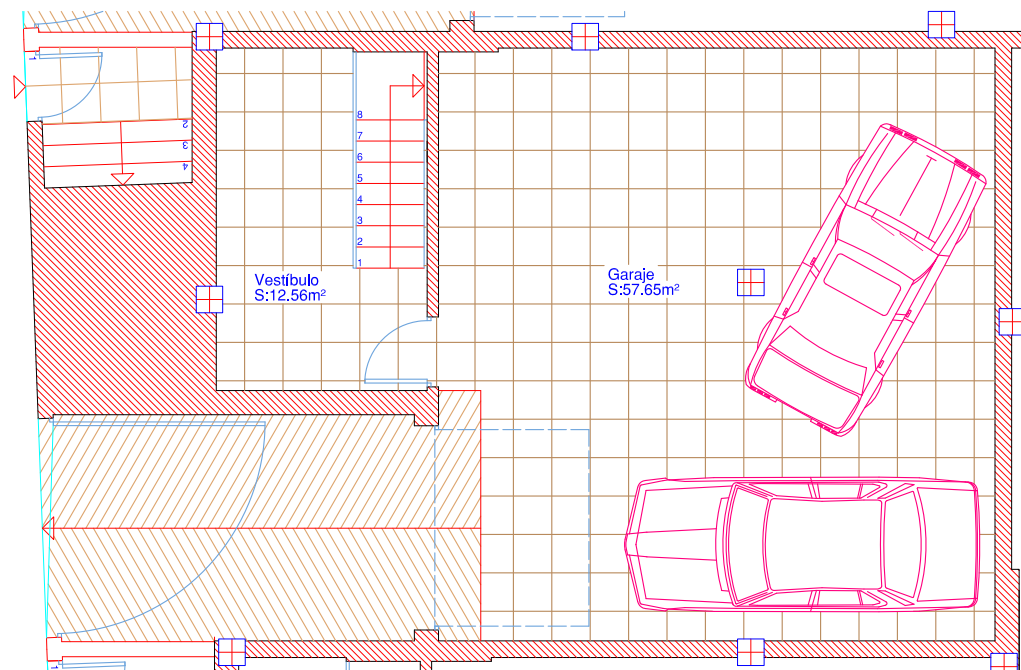
Planta Semisótano
