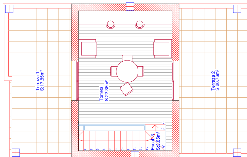
Planta Torreta
