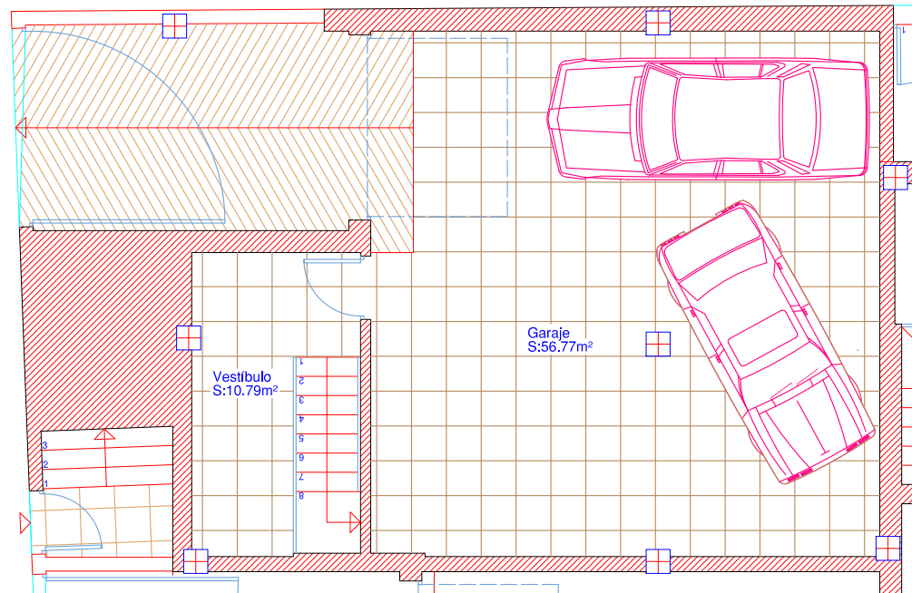
Planta Semisótano
