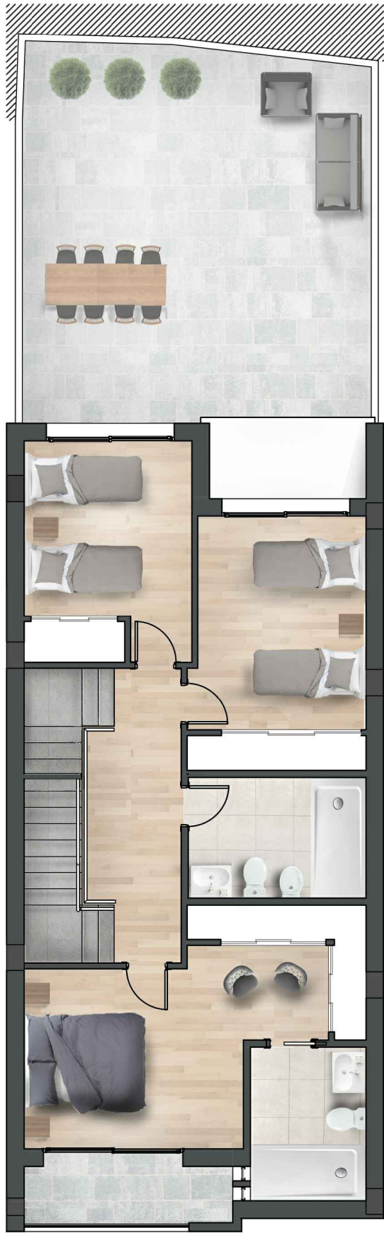
Planta primera
