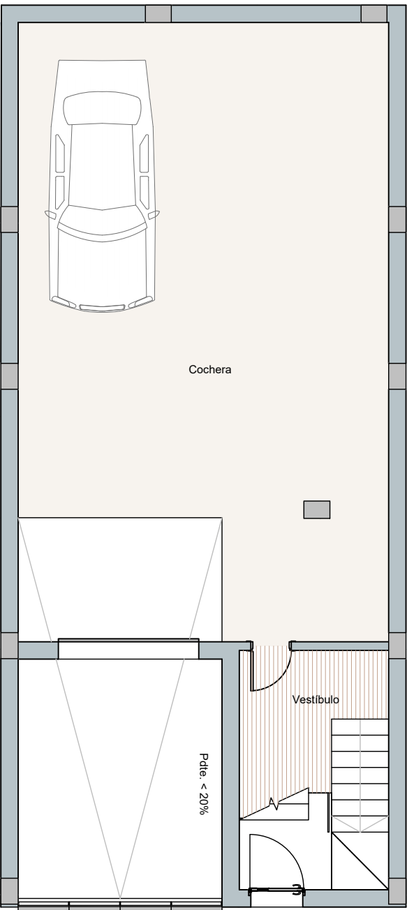
Planta semisótano
