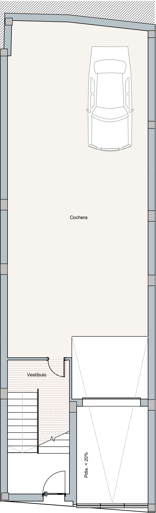
Planta semisótano
