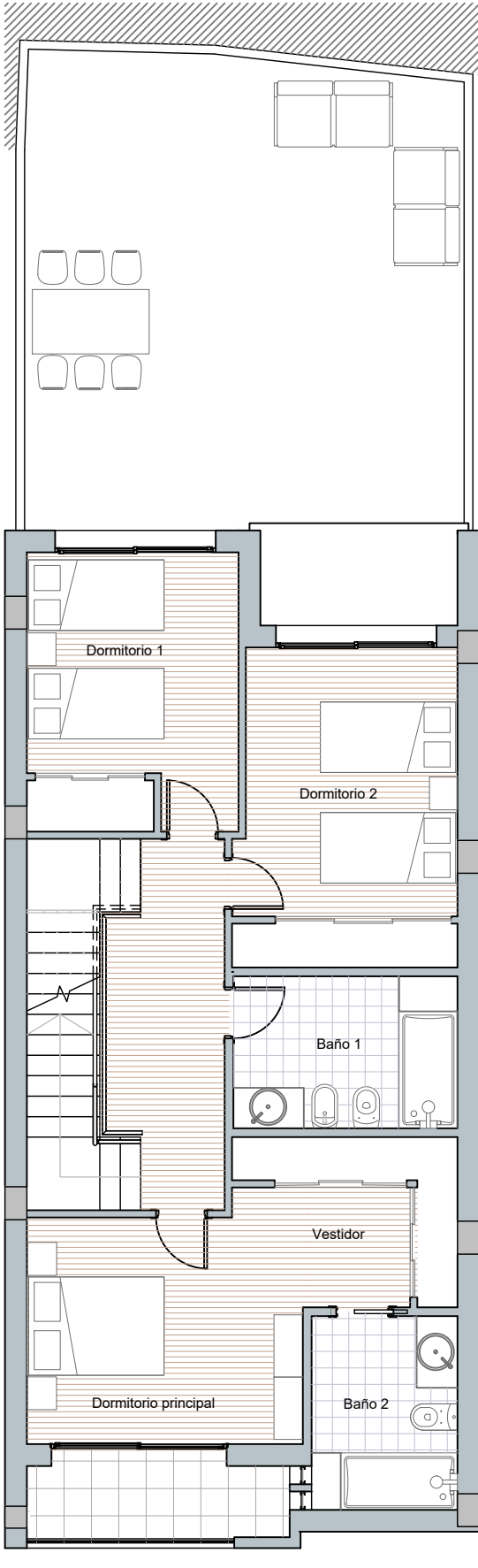
Planta primera
