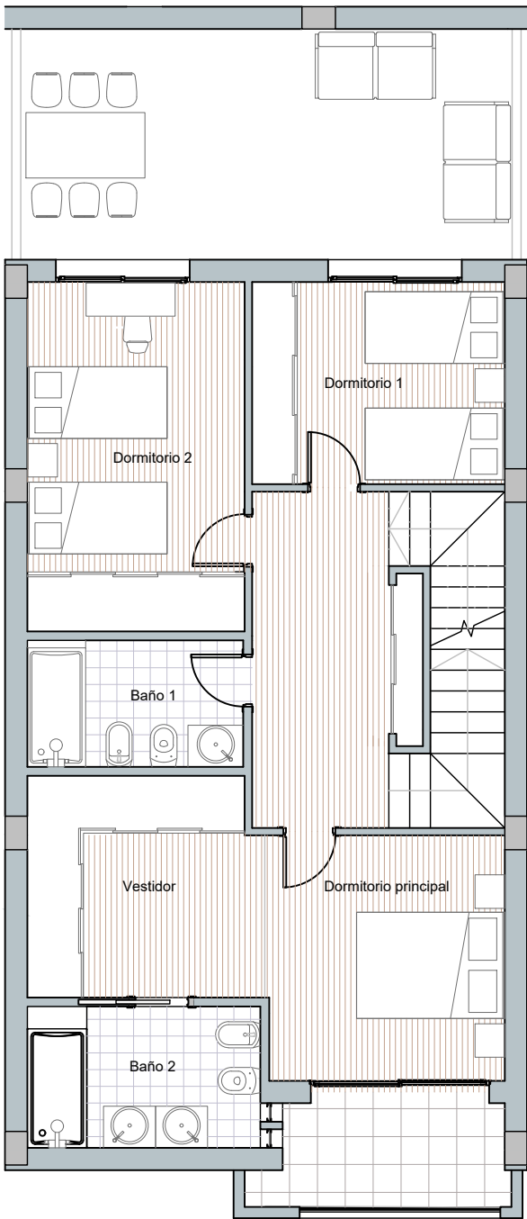
Planta primera
