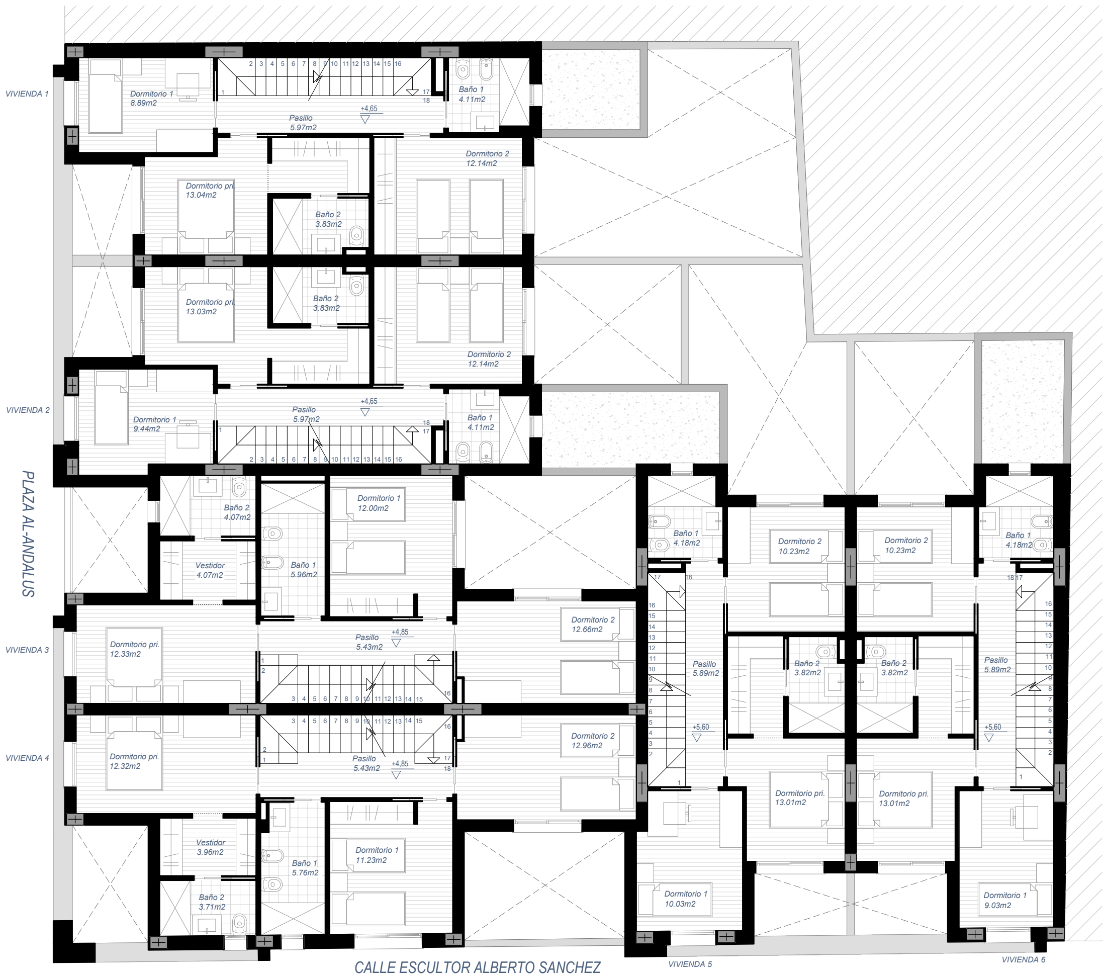
PLANTA PRIMERA
