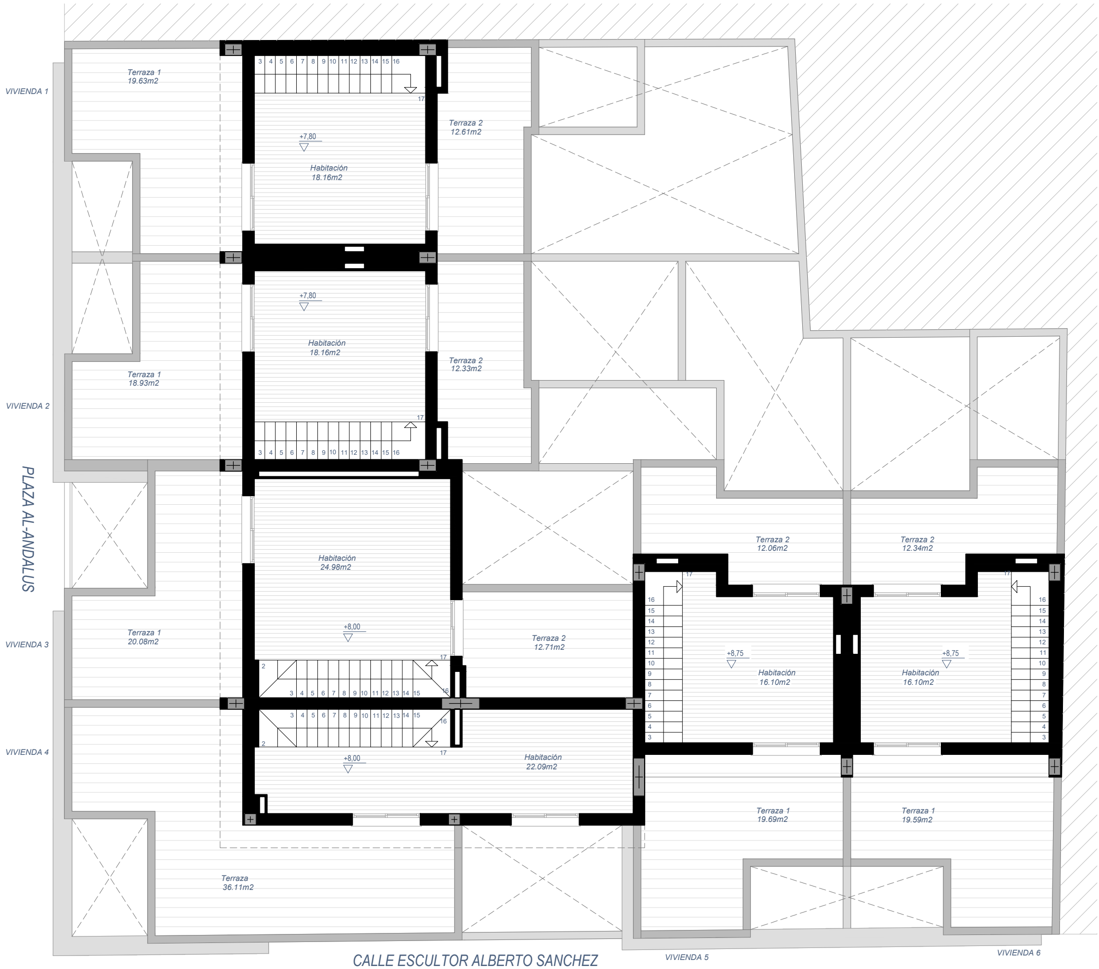
PLANTA TORRETA
